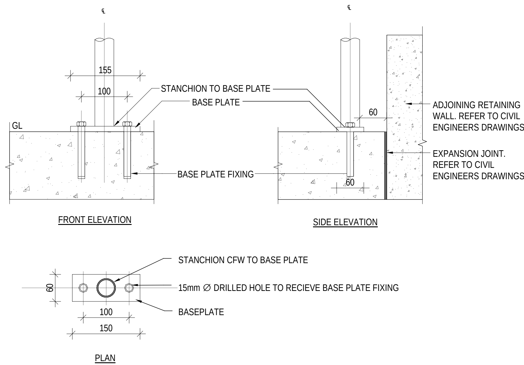
2 HANDRAIL(HR) - BASE PLATE SCALE - 1 : 5
